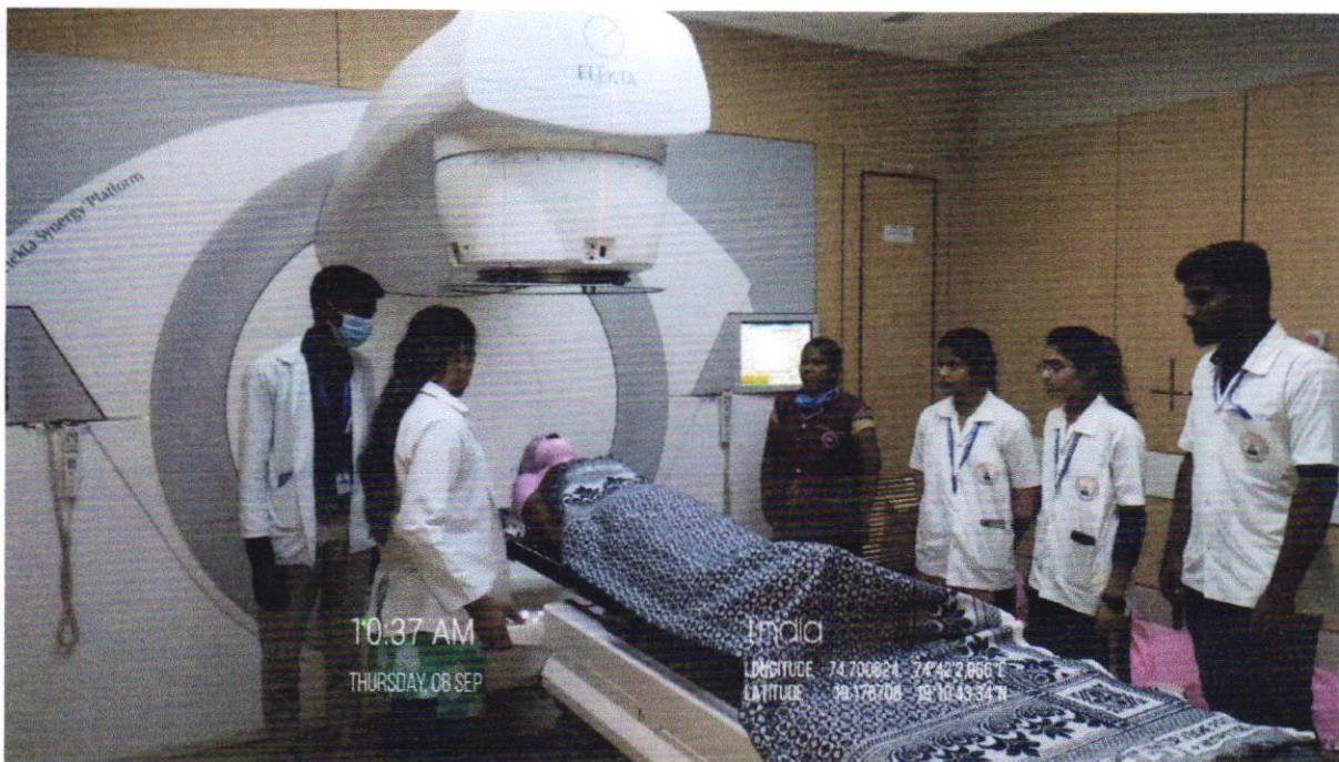
Linear accelerator machine (Double energy Em 6 mv to Em 15 mv)
